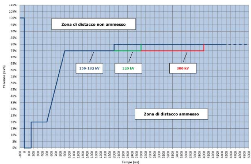
figura 6 – Caratteristica tensione-durata riferita al punto di connessione
